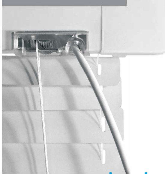
ISOLINE ECO: OVLÁDÁNÍ TYP2 ŠNEK + BOVDEN
